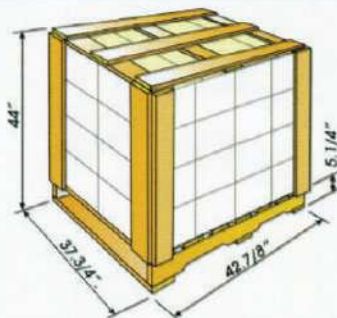
SA pallet Type A (44 Cartons)
