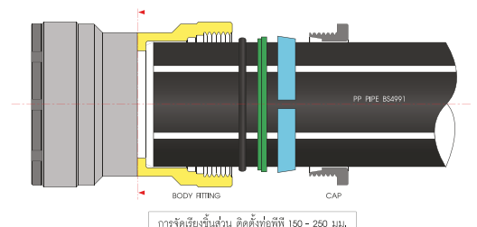
การติดตั้งชิ้นส่วน ติดตั้งท่อพีพี 150 - 250 มม.
