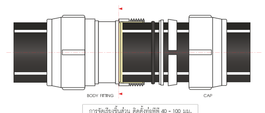
การติดตั้งชิ้นส่วน ติดตั้งท่อพีพี 40 - 100 มม.
